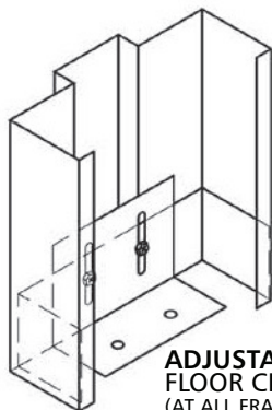
MS (METAL STUD WALLS)
